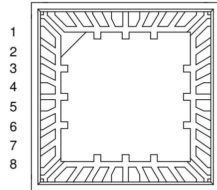
M-QFN32 32L
