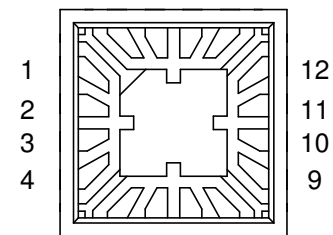
M-QFN16 16L
