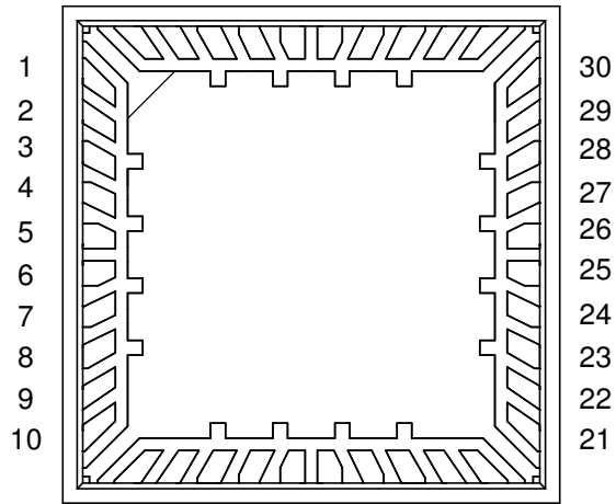
M-QFN40 40L
