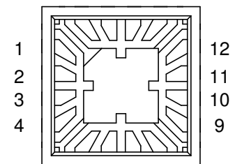
M-QFN16 16L
