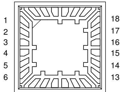
M-QFN24 24L
